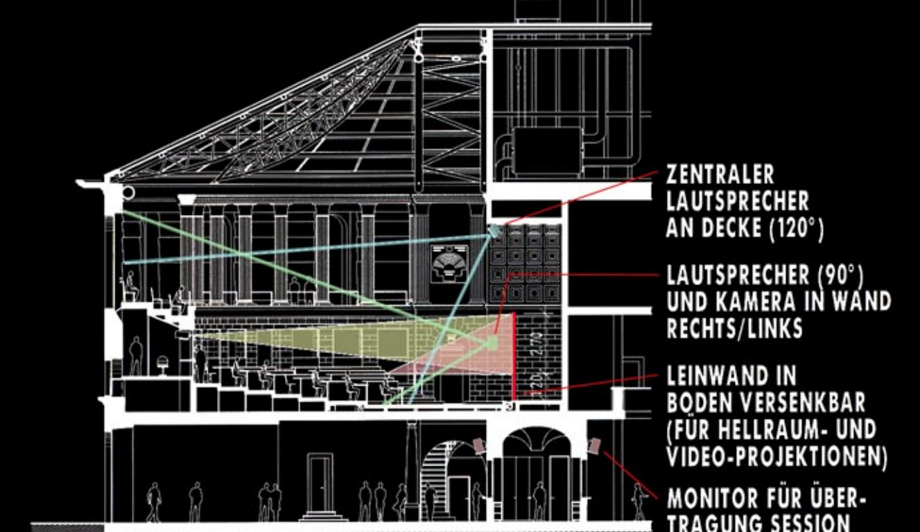
FOYER CAFETERIA/ OFFICE LÄNGSSCHNITT
